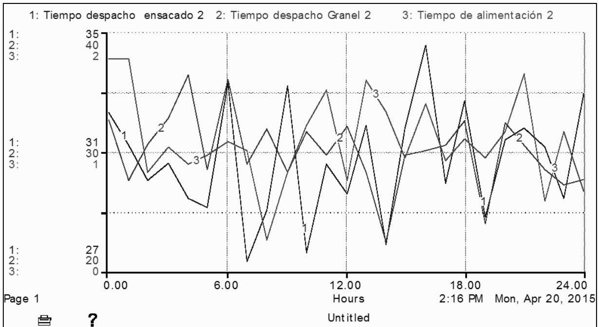
Figura 8. Simulación sistema con Tecnología RFID- Tiempos de despacho granel y ensacado Fuente. Autores
