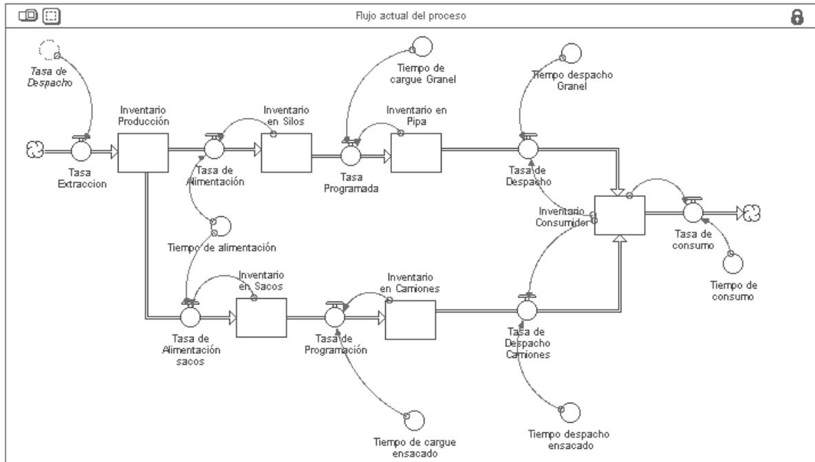
Figura 6. Diagrama Forrester- Simulación sistema actual de operación.
