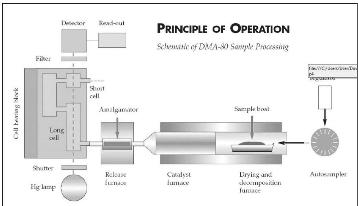
Figura 2. Operación de DMA-80 para la obtención de mercurio en tejido de peces Fuente: Milestone Helping Chemist, 2013
