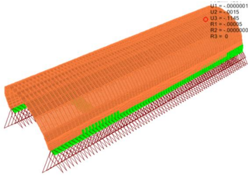
Imagen 7. Deformada Bóveda de Empuje (cm).
