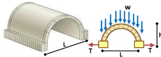
Imagen 2. Diagrama de Cuerpo Libre, Sección transversal Bóveda de Empuje.
