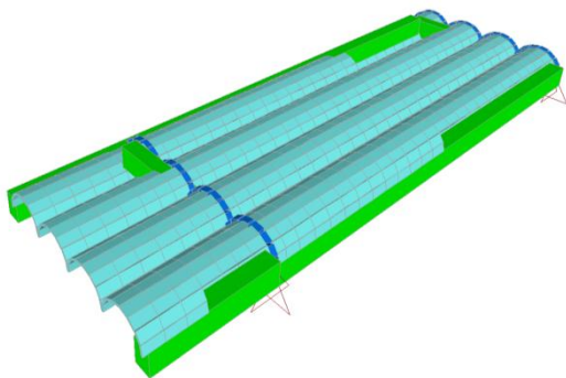
Imagen 8. Modelo Matemático Bóveda tipo Membrana 15x4.8m.
