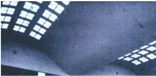
Imagen 5. Cubierta tipo Bóveda en Concreto, sistema de membranas maciza en zonas de concentración de esfuerzos.
