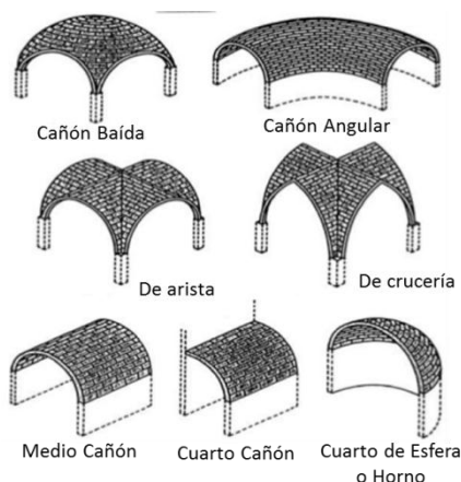
Imagen 1. Bóveda de Empuje, Tipología.
