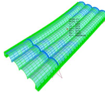
Imagen 9. Deformada Bóveda tipo Membrana (cm).
