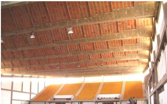
Imagen 22. Bóvedas Plegadas, Coliseo Humberto Perea (Barranquilla, 1961).
