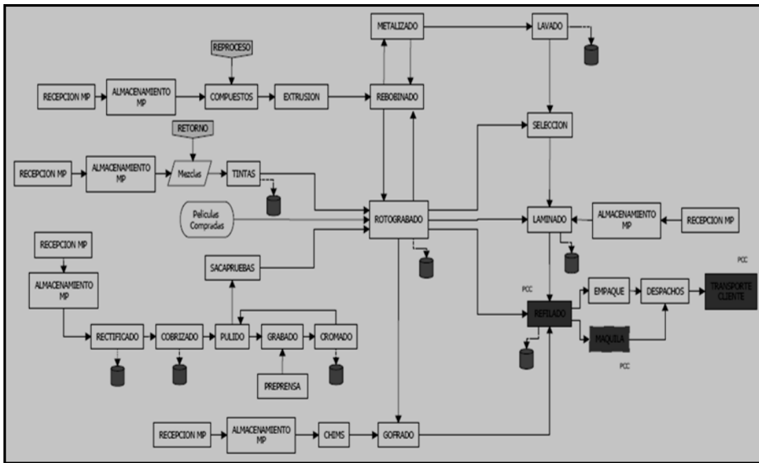
Figura 1. Proceso de elaboración Empaques Plásticos Flexibles
