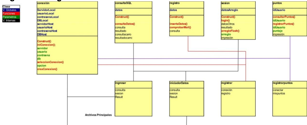
Figura 13. Diagrama de Clases PHP
