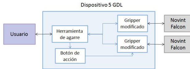
Figura 3.2: Diagrama de bloques dispositivo mecánico 5 GDL
