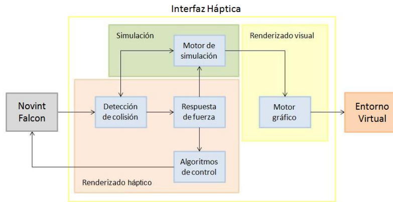
Figura 3.3: Interfaz háptica
