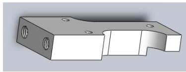
Figura 3.5: Placa horizontal para modificar el gripper del Novint Falcon
