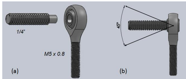
Figura 3.9: Modificación de la rótula. (a) Tornillo mecanizado añadido. (b) Resultado rótula.
