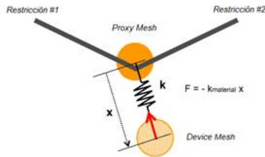
Figura 2.8: Representación de las 2 mallas de la herramienta háptica. Malla Proxy y malla del dispositivo
