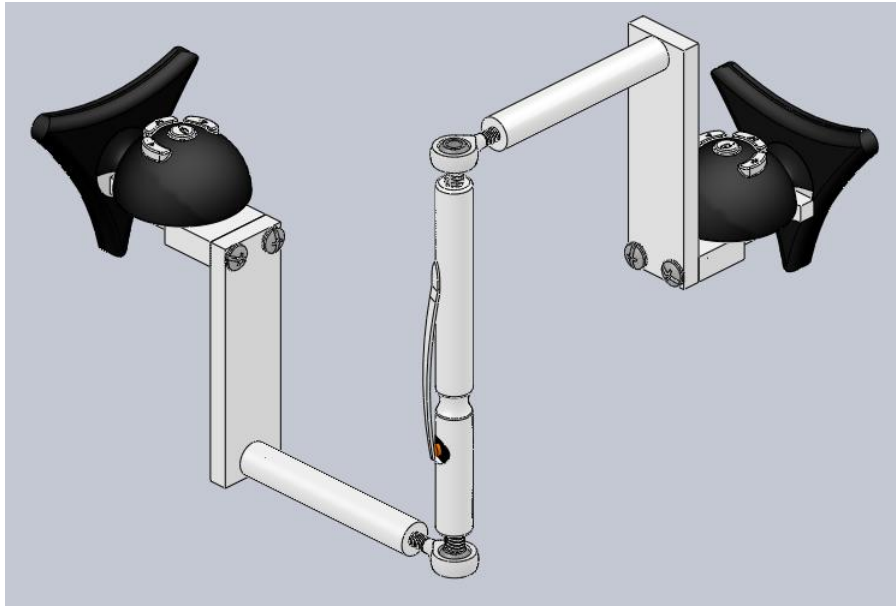
Figura 3.11: Ensamble completo dispositivo 5 GDL.
